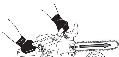
PULL IN / ATTRAZIONE TRACCIÓN / TRACTION
